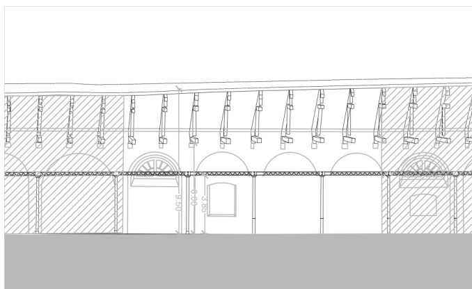
LONG SECTION B-B'
